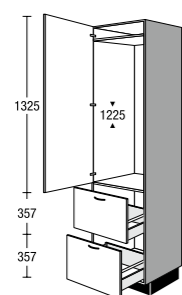
G 122 2A 02 Seitenschrank für Einbaugeräte Tall unit for built-in appliances
