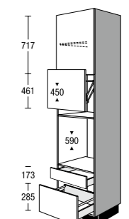
CGMBSA 03 VLQ CGMBSA 03 VLQ Seitenschrank für Einbaugeräte (Abbildung zeigt CGMBSA 03 VLQ) Tall unit for built-in appliances (illustration shows CGMBSA 03 VLQ)
