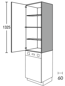
A...133 Aufsatzschrank Top-mounted unit
