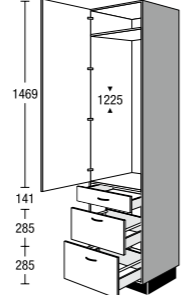
G 122 S2A 03 Seitenschrank für Einbaugeräte Tall unit for built-in appliances
