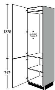
G 122 02 Seitenschrank für Einbaugeräte Tall unit for built-in appliances
