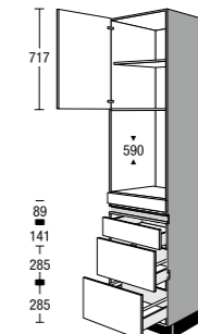
CGBS2A 03 H Seitenschrank für Einbaugeräte Tall unit for built-in appliances
