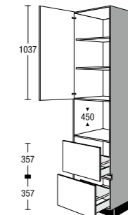
CGM2A 03 H Seitenschrank für Einbaugeräte Tall unit for built-in appliances
