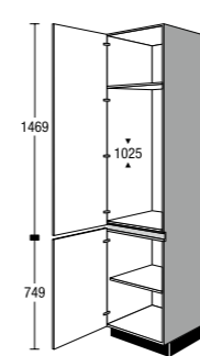
CG 102 03 H Seitenschrank für Einbaugeräte Tall unit for built-in appliances
