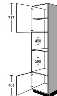
CGMB 03 VQ Seitenschrank für Einbaugeräte Tall unit for built-in appliances
