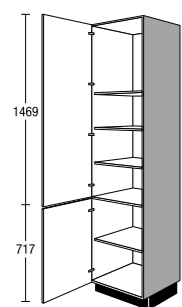
S...03 Seitenschrank Tall unit
