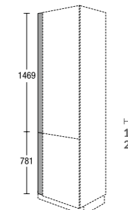
CSPF... 03 V Passleiste für Seitenschrank Infill panel for tall unit
