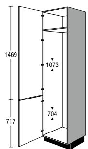
G 178 03 Seitenschrank für Einbaugeräte Tall unit for built-in appliances
