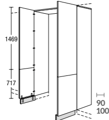
DG... 03 Durchgangstür Access door
