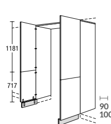
DG... 01 Durchgangstür Access door
