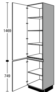
CS...03 H Seitenschrank Tall unit
