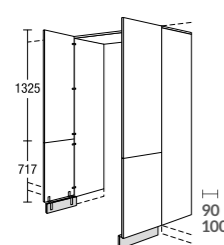
DG... 02 Durchgangstür Access door
