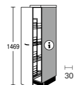
SA... 148 EP Apotheker-Highboard mit Dämpfung Pull-out larder highboard with cushioning
