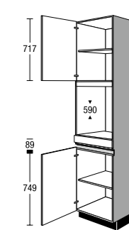
CG B 03 H Seitenschrank für Einbaugeräte Tall unit for built-in appliances
