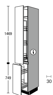
CSA...03 H CSA...03 HP Apotheker-Seitenschrank mit Dämpfung Pull-out tall unit with cushioning
