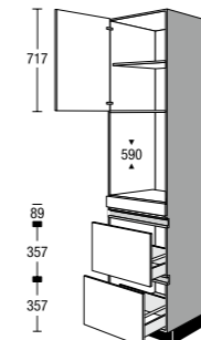
CG B2A 03 H Seitenschrank für Einbaugeräte Tall unit for built-in appliances
