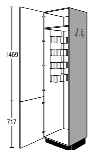
S...03 B Seitenschrank für Besen Tall broom cupboard
