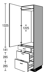
G 122 S2A 02 Seitenschrank für Einbaugeräte Tall unit for built-in appliances
