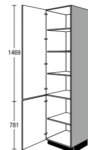
CS...03 V Seitenschrank Tall unit
