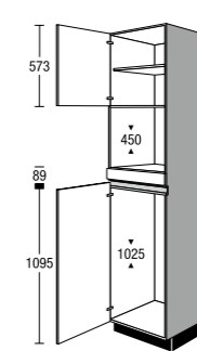
CG 102 M 03 H6 Seitenschrank für Einbaugeräte Tall unit for built-in appliances
