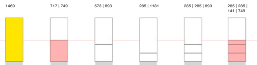
Seitenschrank 2195 mm H03 Linienführung Tall unit 2195 mm H03 line layout
