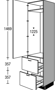
G 122 2A 03 Seitenschrank für Einbaugeräte Tall unit for built-in appliances
