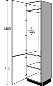
G 122 03 Seitenschrank für Einbaugeräte Tall unit for built-in appliances
