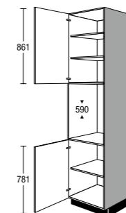
CGB 03 V Seitenschrank für Einbaugeräte Tall unit for built-in appliances
