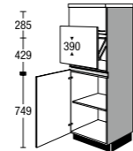
G122 148 E Highboard für Einbaugeräte Highboard for built-in appliances
