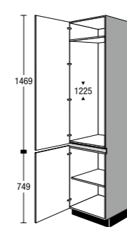
CG 122 03 H Seitenschrank für Einbaugeräte Tall unit for built-in appliances
