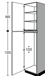
CG 122 03 H9 Seitenschrank für Einbaugeräte Tall unit for built-in appliances
