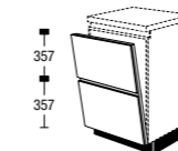
CTGV 60 M2 Frontplatte mit geteilter Front und Griffprofil Front plate with split front and handle profile
