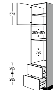
CGMBSA 03 HX Seitenschrank für Einbaugeräte Tall unit for built-in appliances
