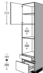
CGMBSA 03 H Seitenschrank für Einbaugeräte Tall unit for built-in appliances
