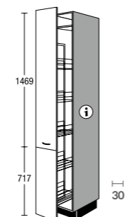
SA...03 P Apotheker-Seitenschrank mit Dämpfung Pull-out tall unit with cushioning
