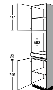
CSA 30 03 V CSA 30 03 VP Apotheker-Seitenschrank mit und ohne Dämpfung Pull-out tall unit with and without cushioning
