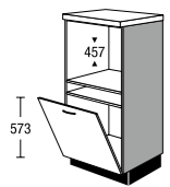
GMG 104 X Highboard für Einbaugeräte Highboard for built-in appliances
